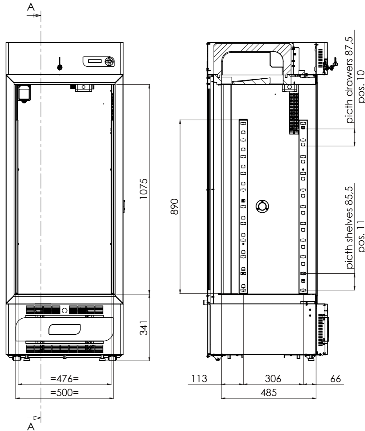
SECTION A-A
