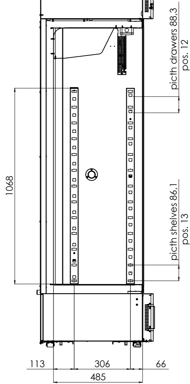
SECTION A-A
