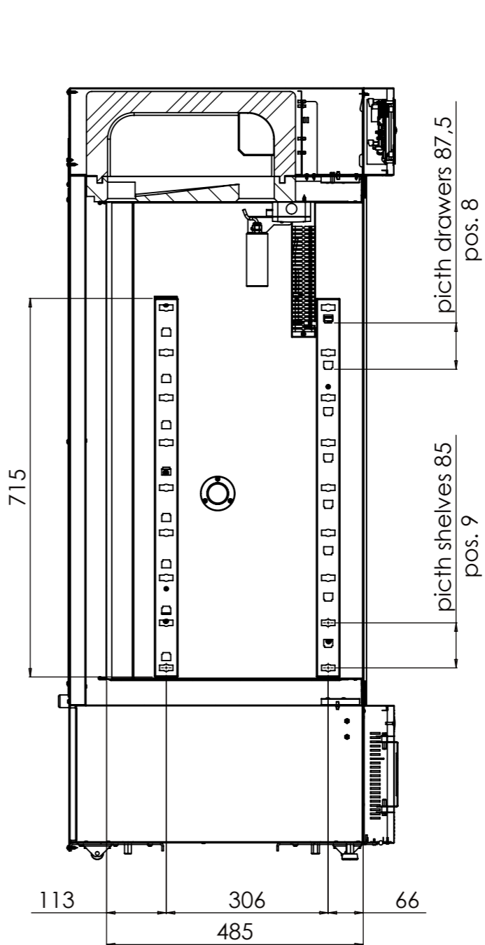
SECTION A-A
