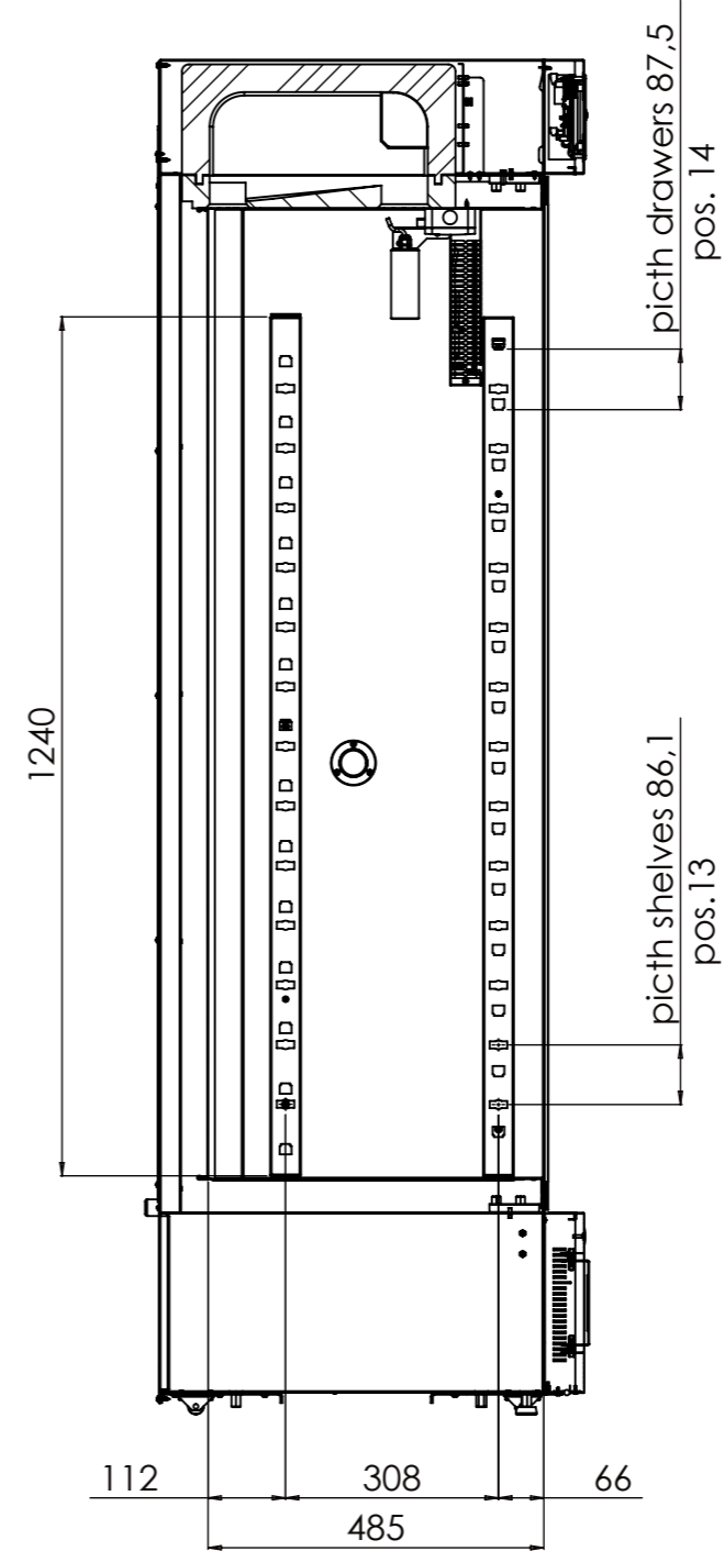
SECTION A-A
